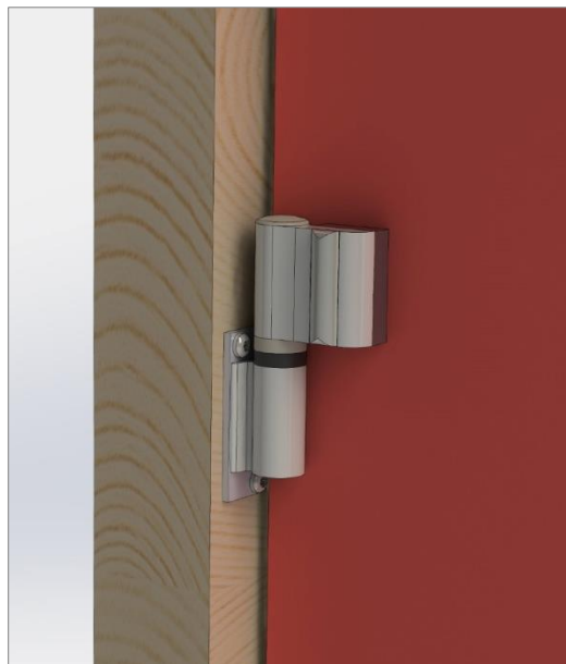
Détail : montage de la paumelle cabine sur l' huisserie
